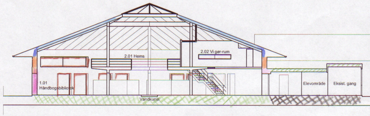
Tværsnit A-A 1:200
