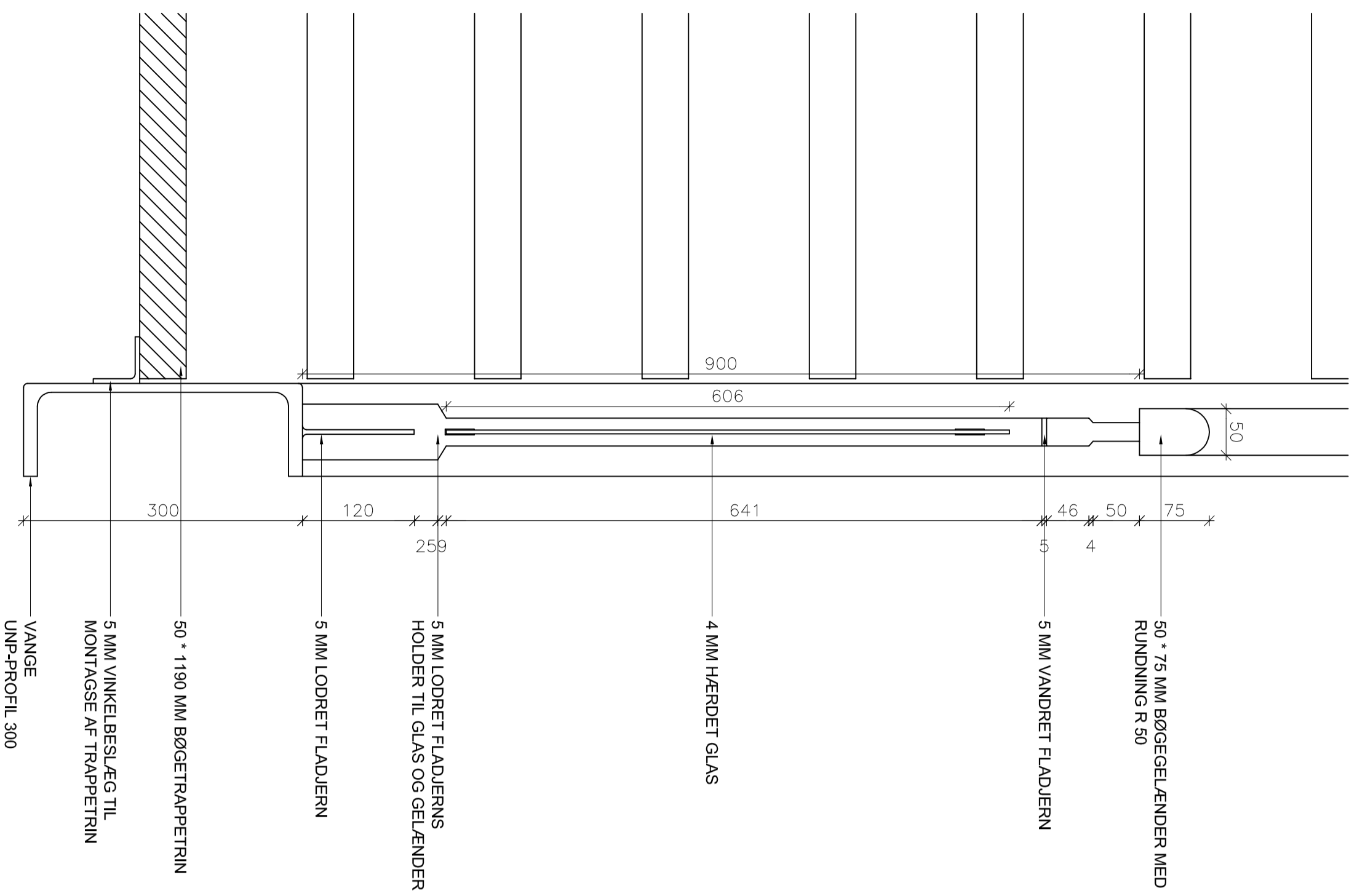
1:5 SNIT A:A
