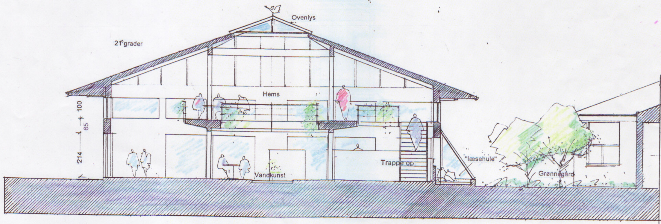
TVÆRSNIT A-A Ca. 1:100
